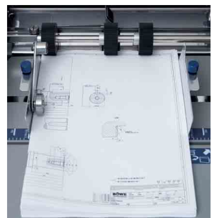
Versetzbare Einzugswalze (links) für einen optimalen Einzug beim Kreuzfalz
